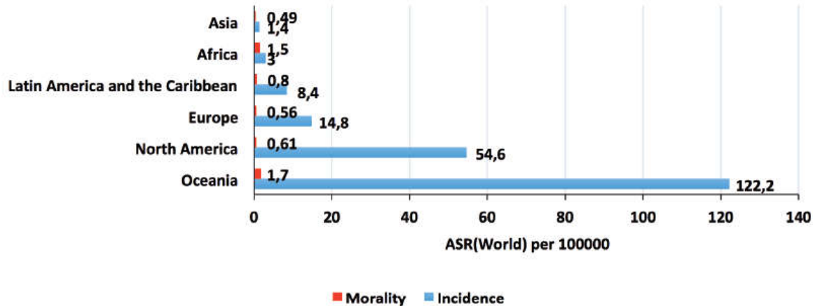
Fig.7. Incidența și mortalitatea pentru melanomul malign la nivel mondial
